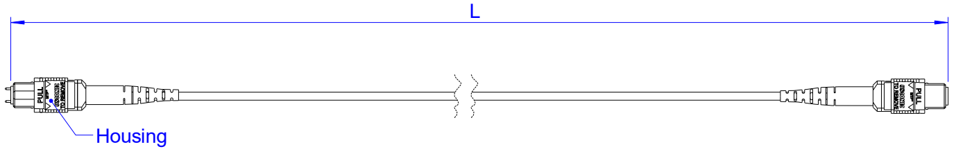
图 2.1 MTP-MTP 跳线
