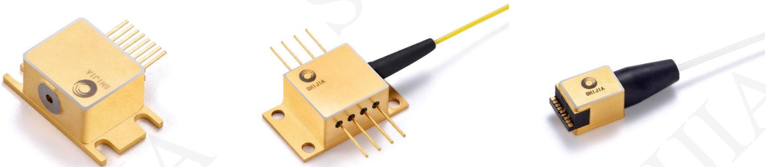
不同类型封装结构
