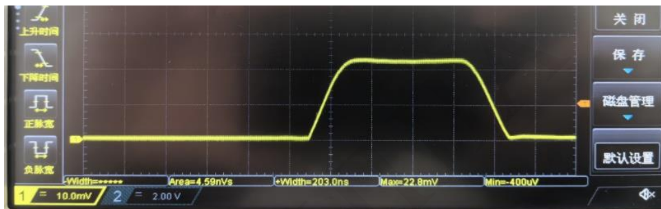
200ns 脉冲
