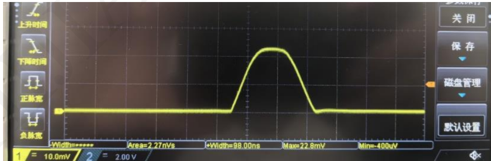
100ns 脉冲
