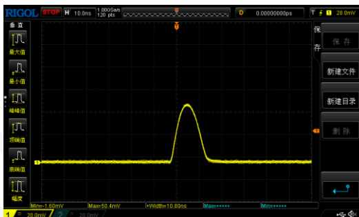
10ns 脉冲
