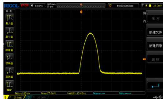
15ns 脉冲
